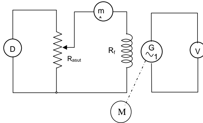
Gambar .2 Rangkaian pengujian beban nol
