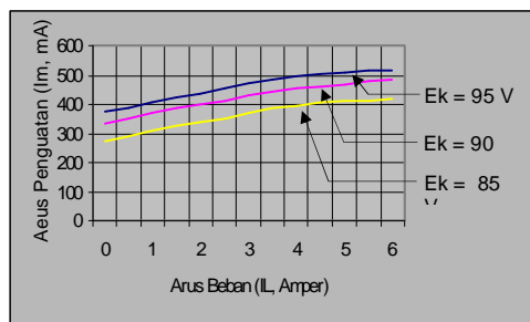
Gambar 7 Kurva Karakteristik Pengaturan
