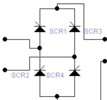
Gambar 2 Penyearah terkontrol
