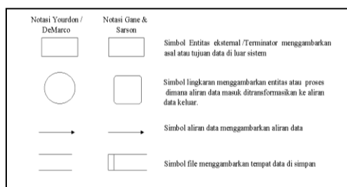
Gambar 1. Simbol DFD
