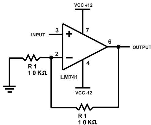
Gambar 3. Rangkaian Op-Amp
